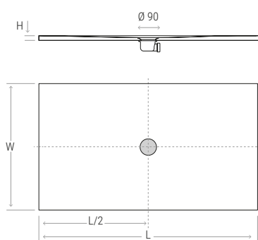
Rechteckig (Zentrierter Ablauf)
